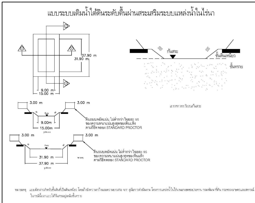
รูปที่ 5-4 ตัวอย่างแบบเติมน้ำผ่านสระเสริมระบบแหล่งน้ำในไร่นา
