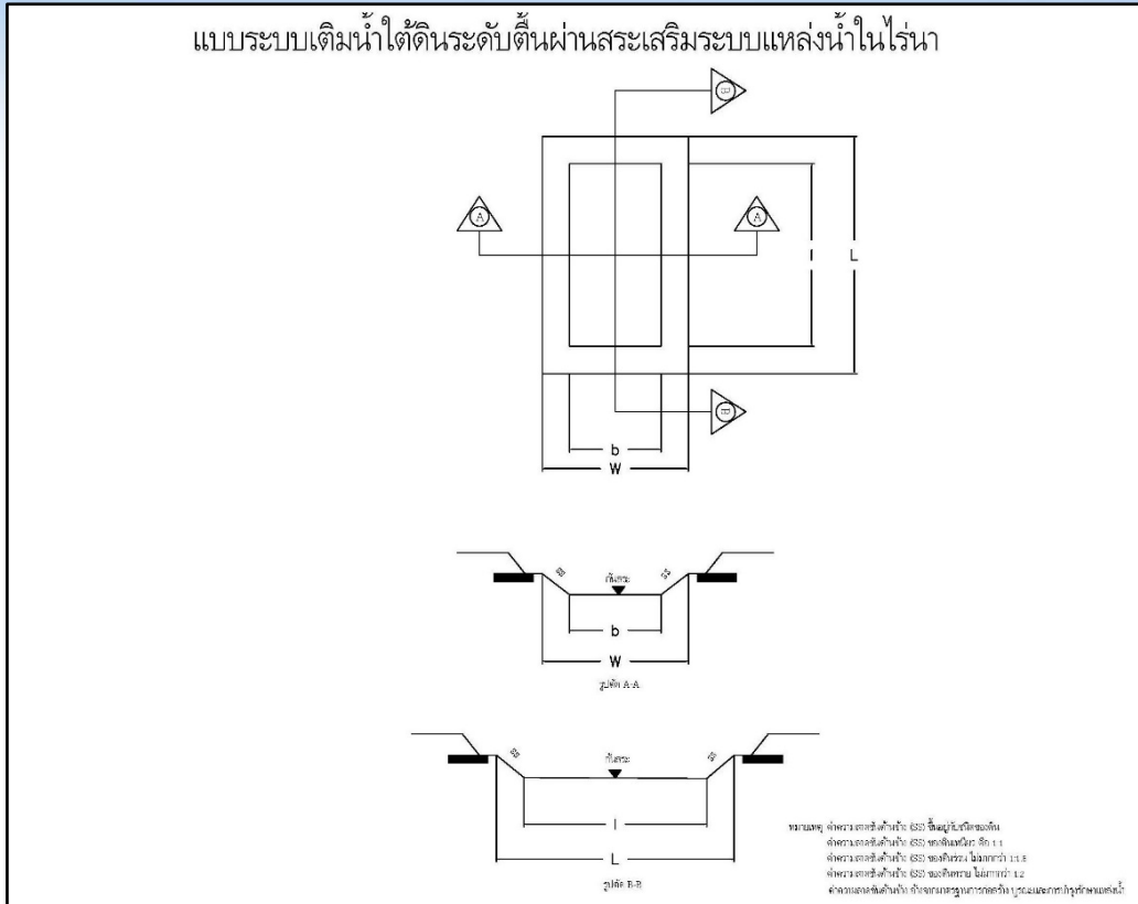
รูปที่ 5-3 แบบเติมน้ำผ่านสระเสริมระบบแหล่งน้ำในไร่นา
