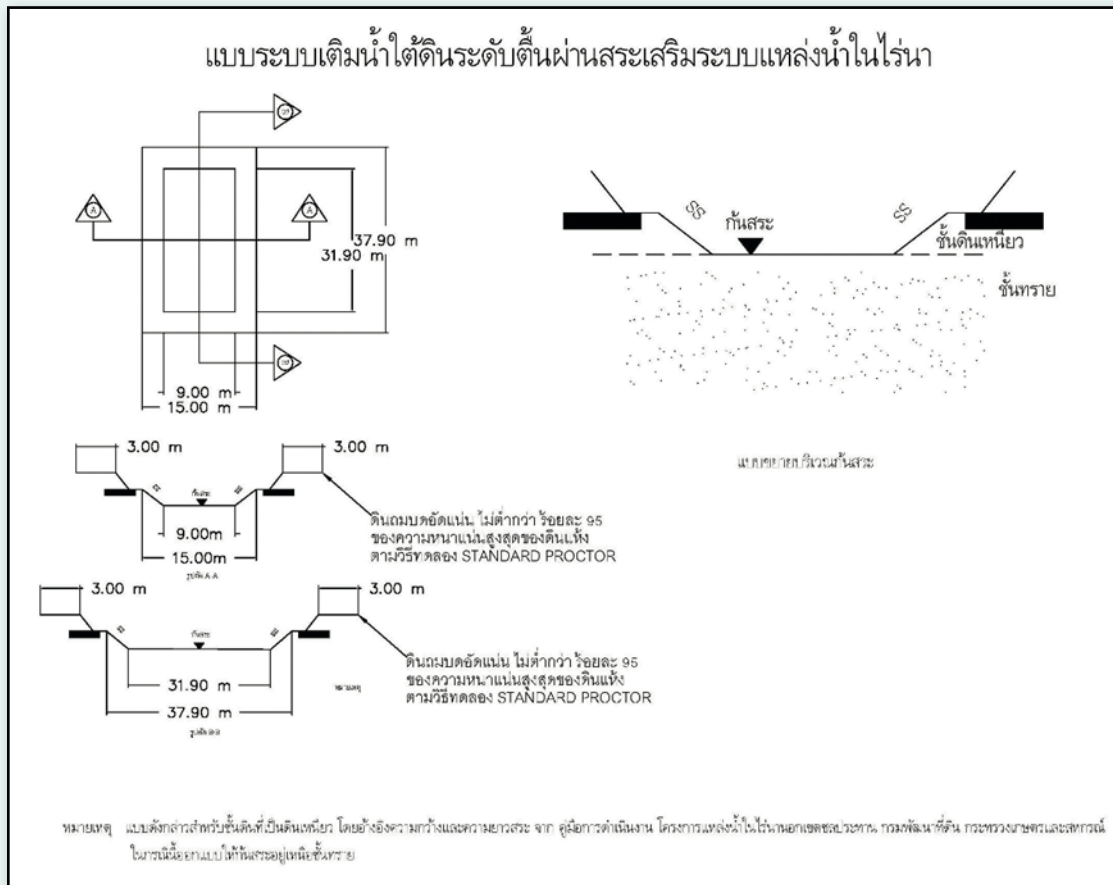
รูปที่ 5.2 ตัวอย่างแบบระบบเติมน้ำใต้ดินระดับต้นผ่านเสริมระบบแหล่งน้ำในไร่นา (ต่อ)
