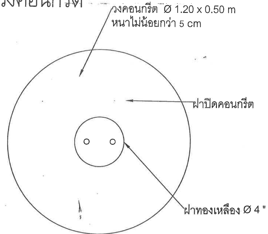
แบบบ่อวงคอนกรีตด้านบน
