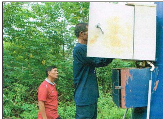
ภาพถ่ายซ่อมแซมระบบประปาบาดาล
