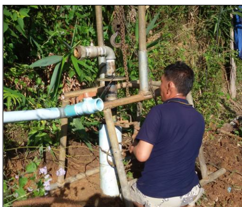
ภาพถ่ายการซ่อมแซมบ่อน้ำบาดาล
