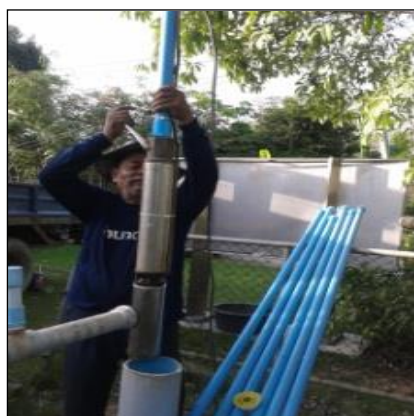
ภาพถ่ายเปลี่ยนเครื่องสูบน้ำ
