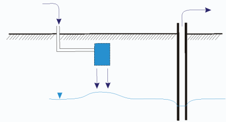
8) สระเติมน้ำ (Infiltration Pond)
