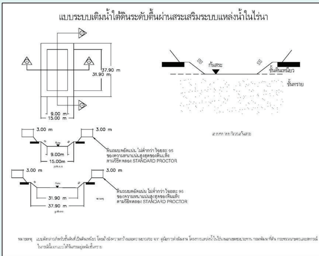
รูปที่ 5.2 ตัวอย่างแบบระบบเติมน้ำใต้ดินระดับตื้นผ่านสระเสริมระบบแหล่งน้ำในไร่นา (ต่อ)
